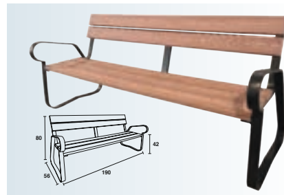
Modelo 18 BILBAO
