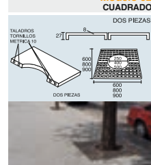
Modelo 02 CUADRADO
