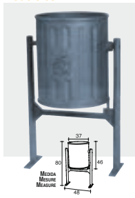
PAPELERA Modelo 08
