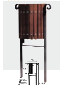
PAPELERA Modelo 13
